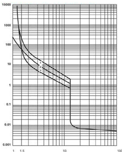
1. 3-polige belasting in koude toestand 2. 2-polige belasting in koude toestand 3. 3-polige belasting in warme toestand
